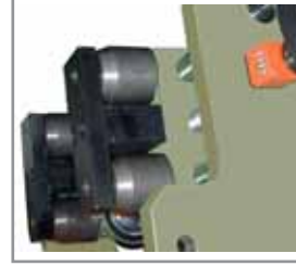
Guidanastri con indicatore numerico Entry guides with numeri- cal gauge
